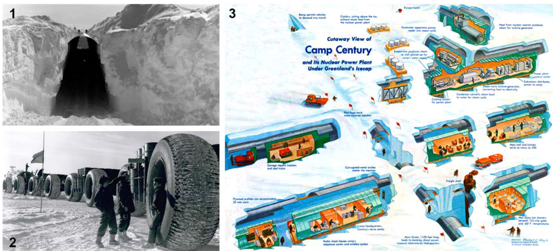
Figura 01-1: Pictorial Parade/Archive Photos/Getty Images. Uma visão da rampa de acesso principal para o acampamento permanente Camp Century. Anos 50. 1 fotografia. Figura 01-2: Zumapress. Um transportador logístico de carga deixa suprimentos no Camp Century . 1959. 1 fotografia. | Figura 01-3: Robert C. Magie/National Geographic. Cutaway of Camp Century and Its Nuclear Power Plant Under Greenland's Icecap (Vista cortada do Camp Century e sua planta nuclear sob a camada de gelo da Groenlândia). 1962. 1 ilustração.
